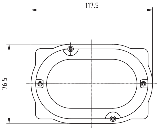
正视图
