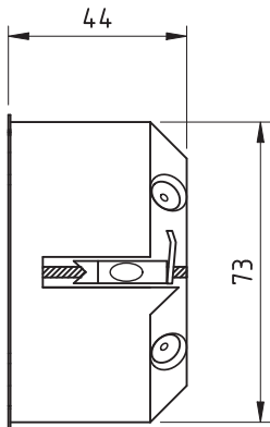
侧视图
