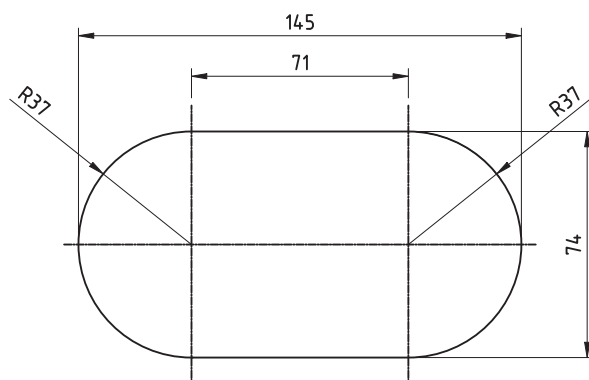
开孔图
